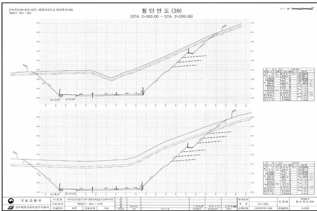
【그림 62-4】 표준횡단면도
