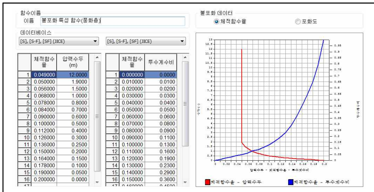
【그림 62-15】 압력수두-채적함수물(포화도)-투수계수비 함수
